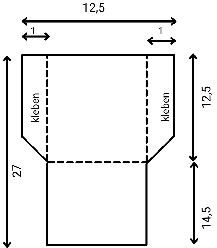
Schnittzeichnung Tasche
